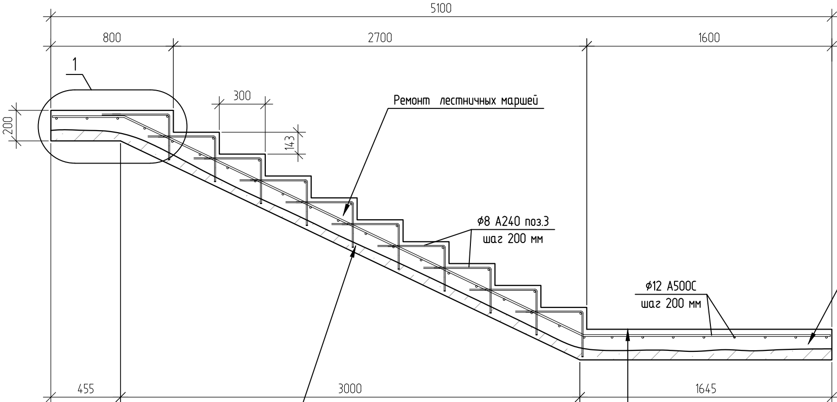
Армирование 1-1
