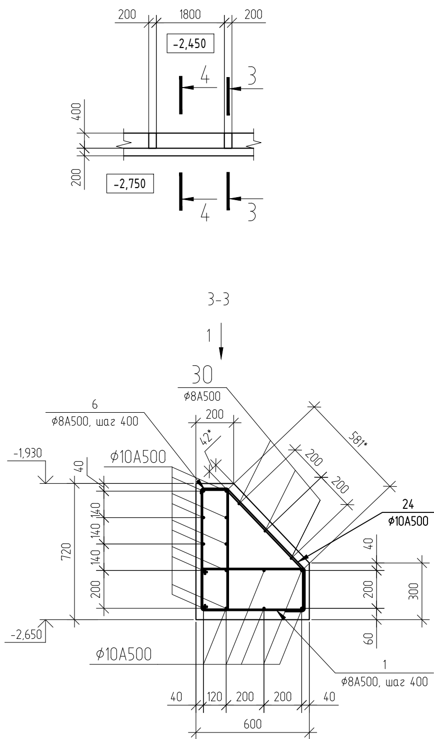
Подпорная стена ПС-1.5 (фрагмент)
