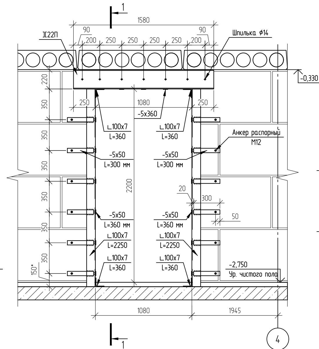
Схема устройства усиления проема Пр-1
