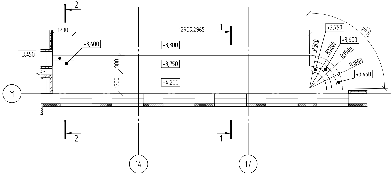
Зрительная трибуна Фрагмент плана на отм. +3.300 в осях 13-21/М
