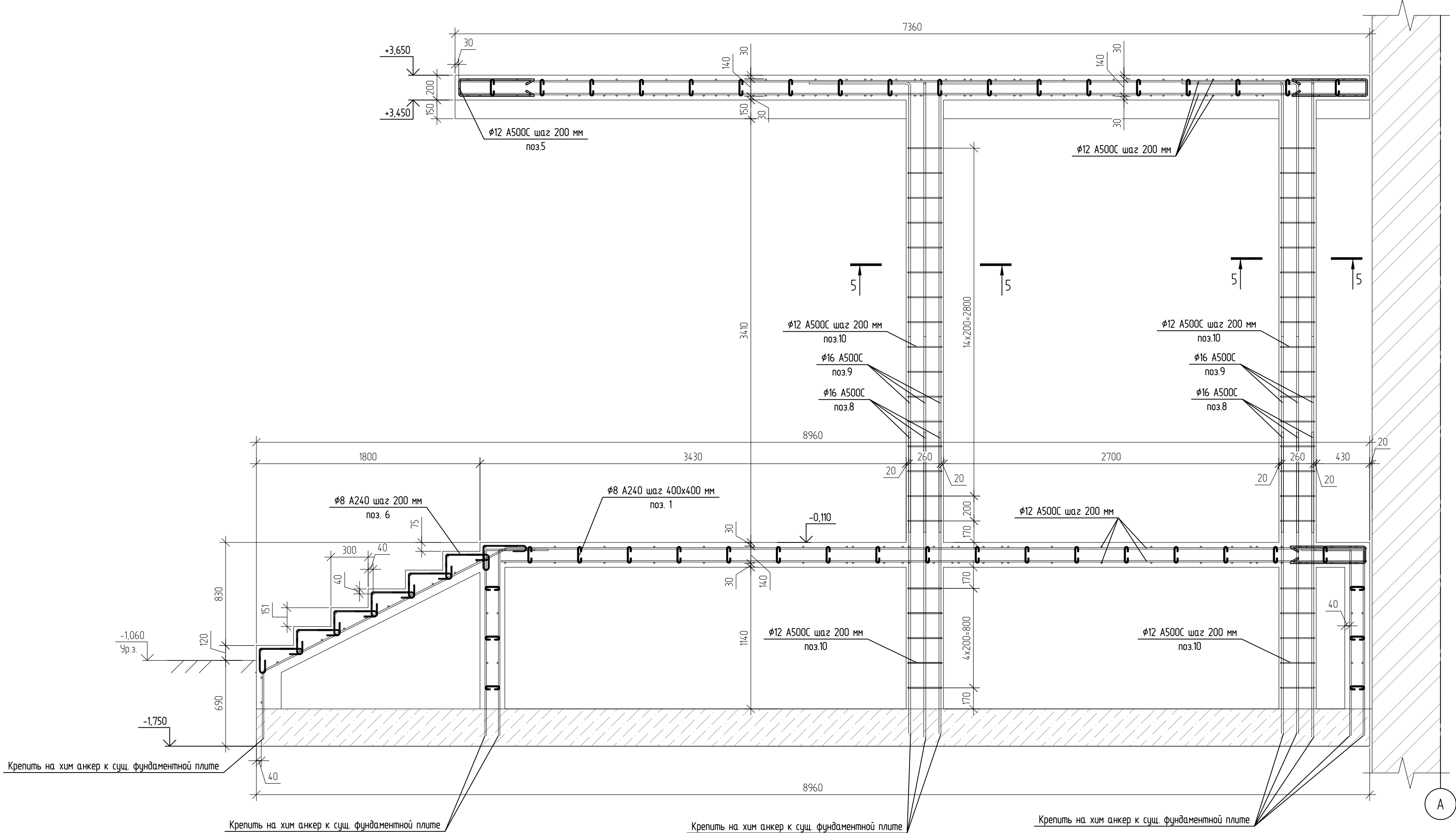
Армирование. Разрез 2-2
