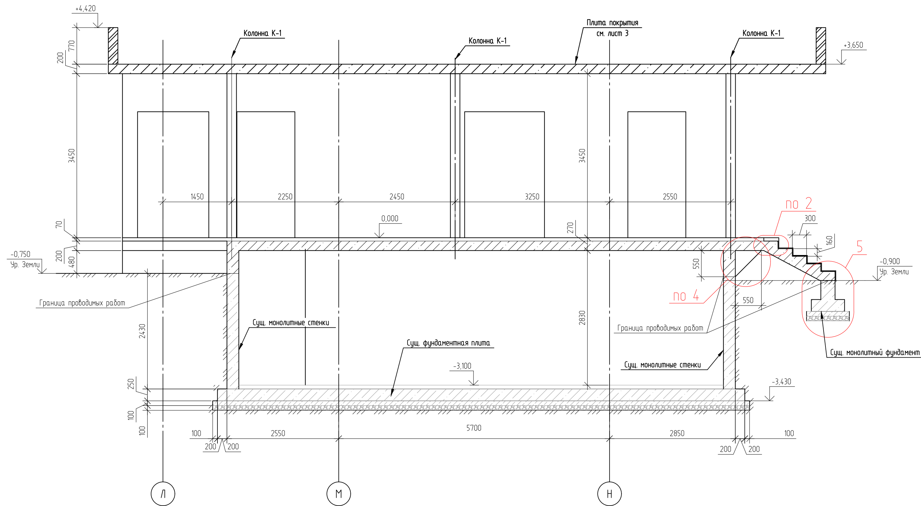
Разрез 3-3
