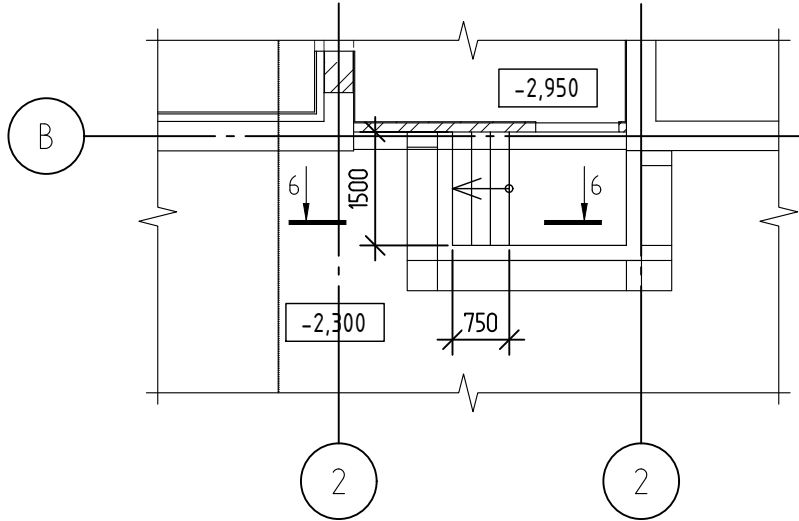
Схема расположения лестницы Л-4
