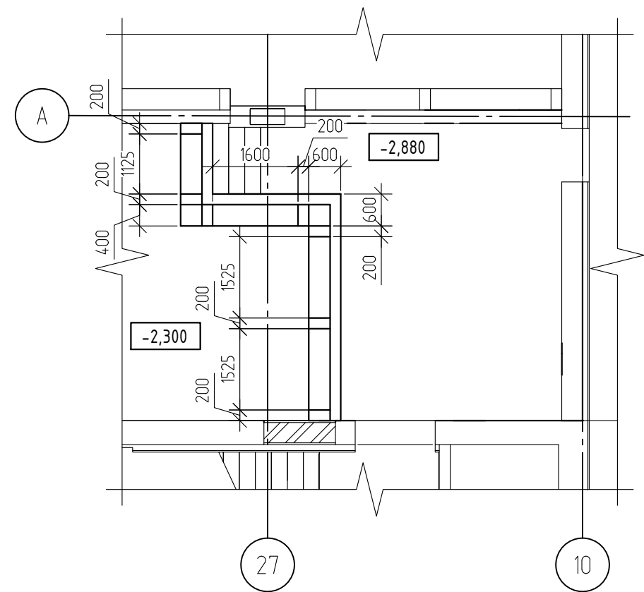
Подпорная стена ПС-1.9
