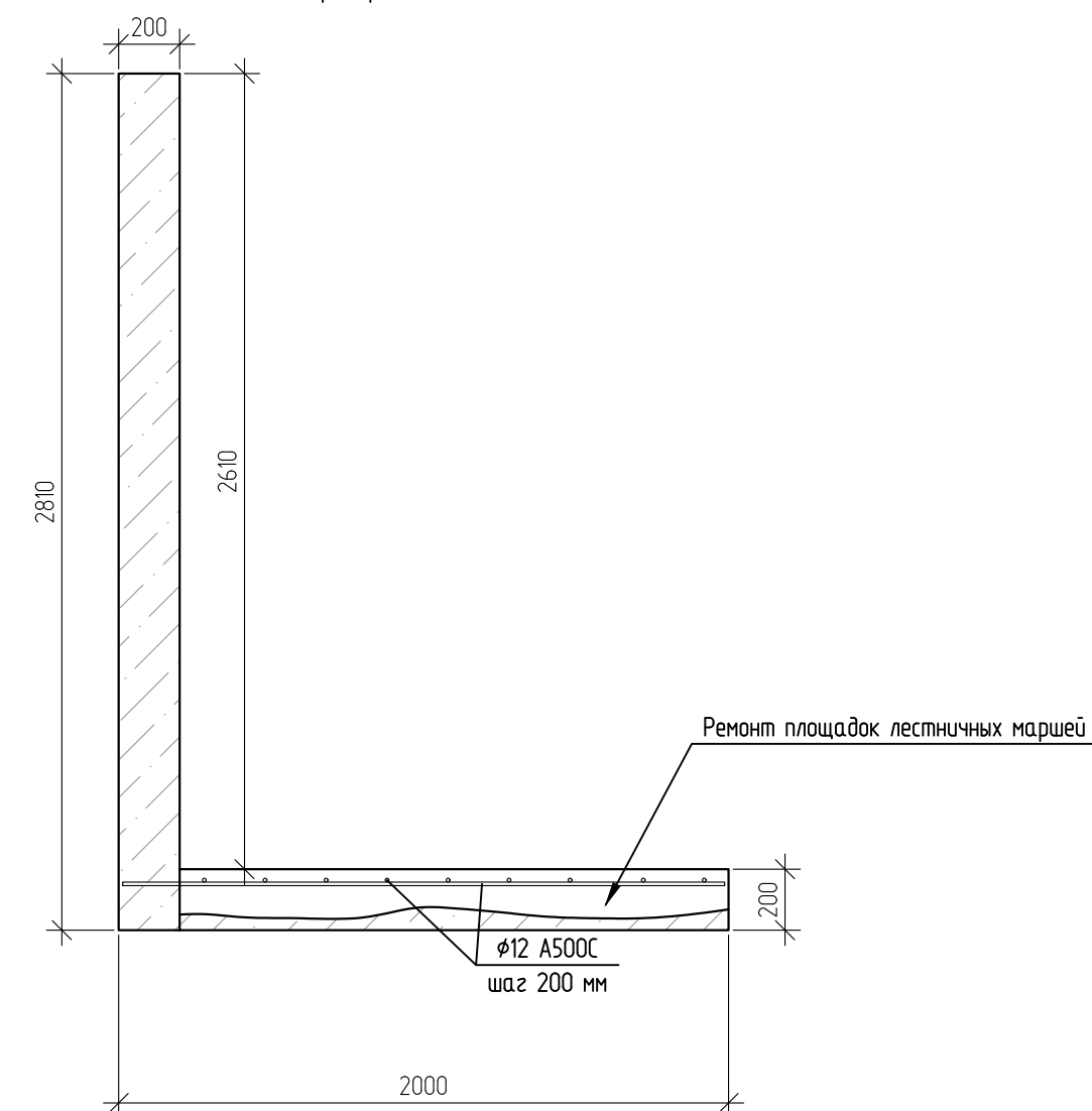
Армирование 2-2
