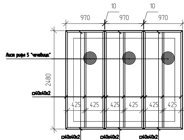
Устройство крышки прямка
