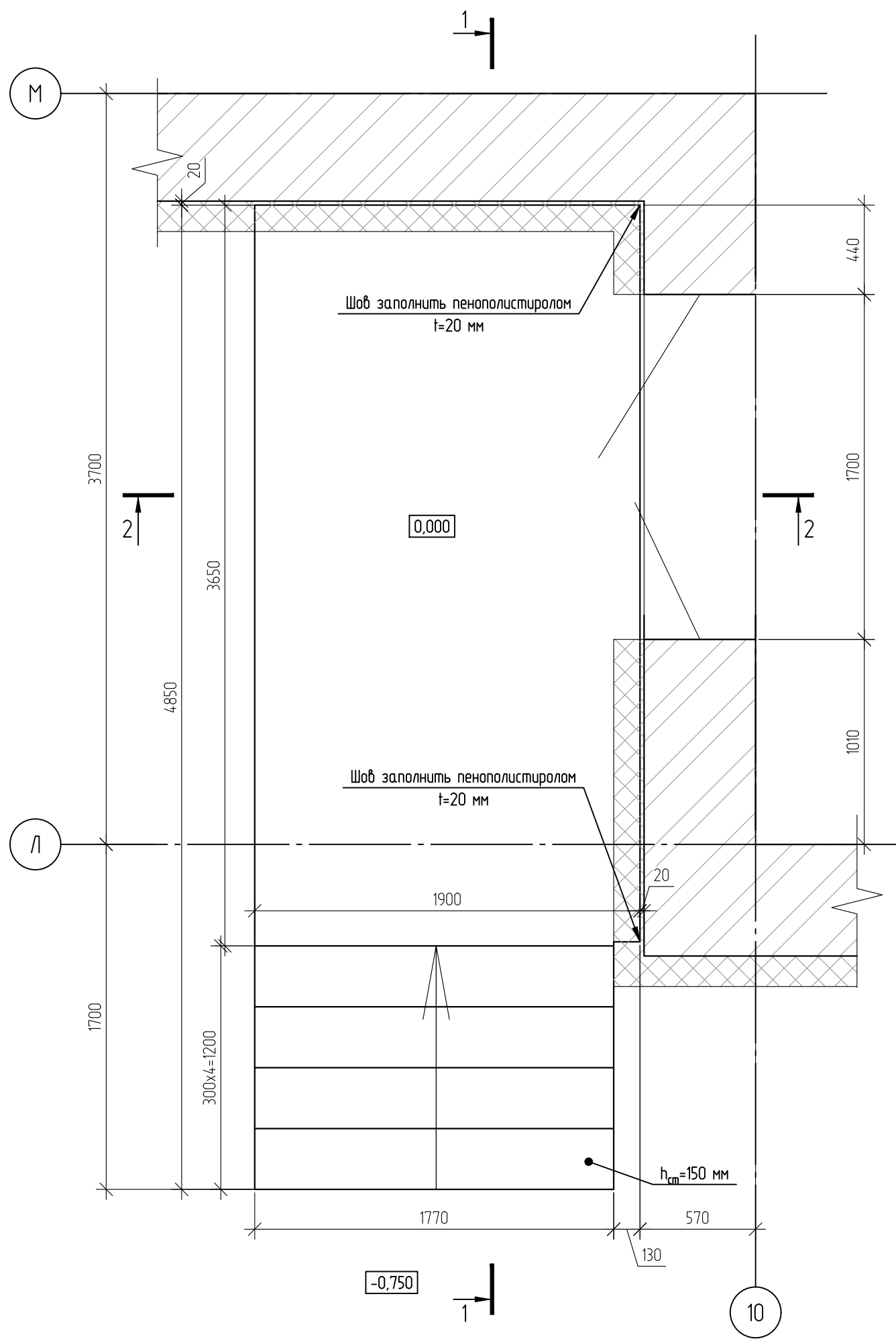
Схема устройства входа в осях "10/Л-М"
