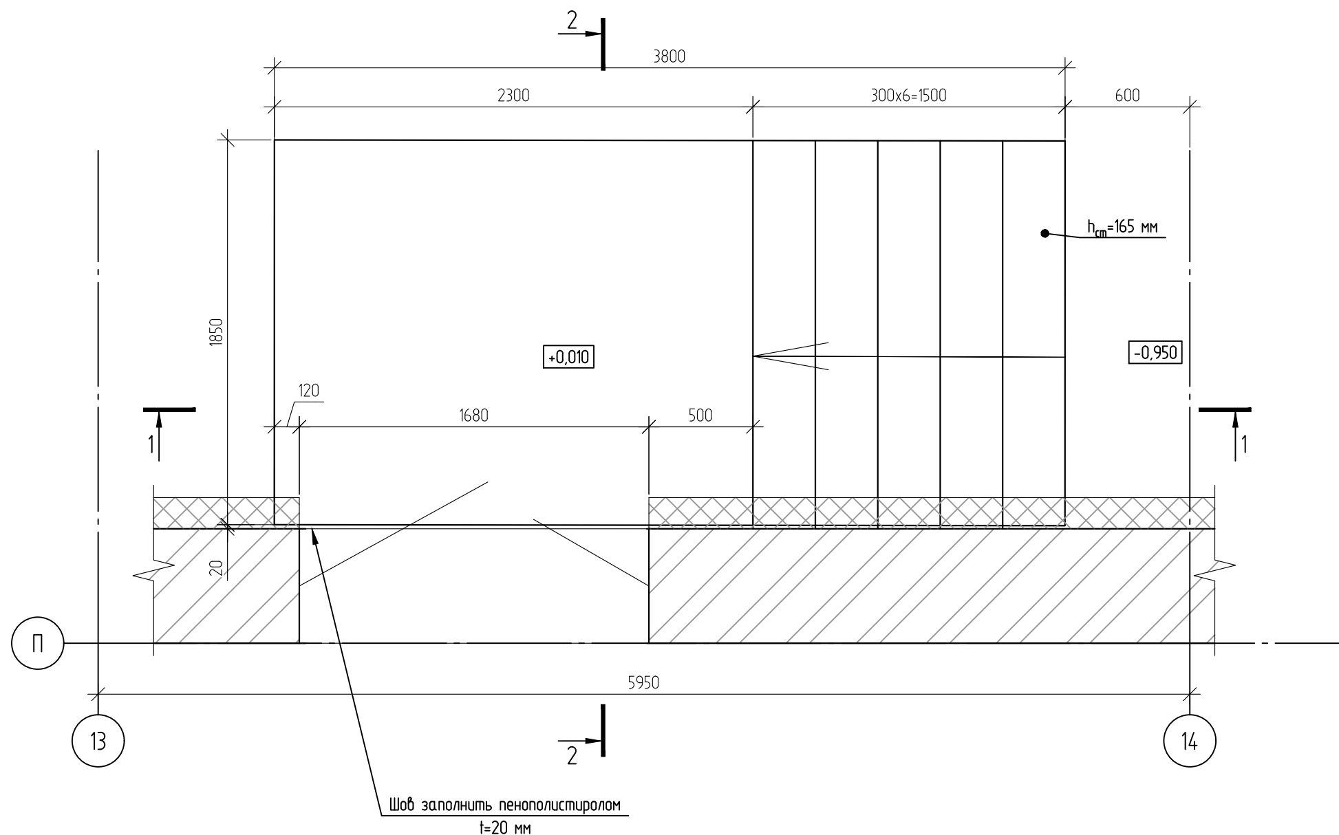
Схема устройства входа в осях "13-14/П"
