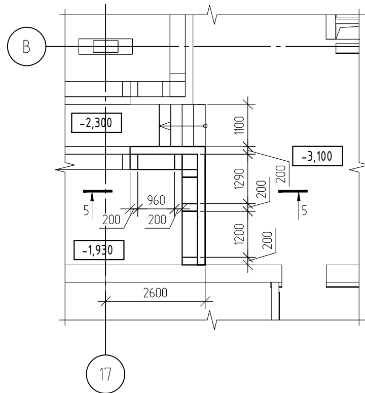
Подпорная стена ПС-1.7
