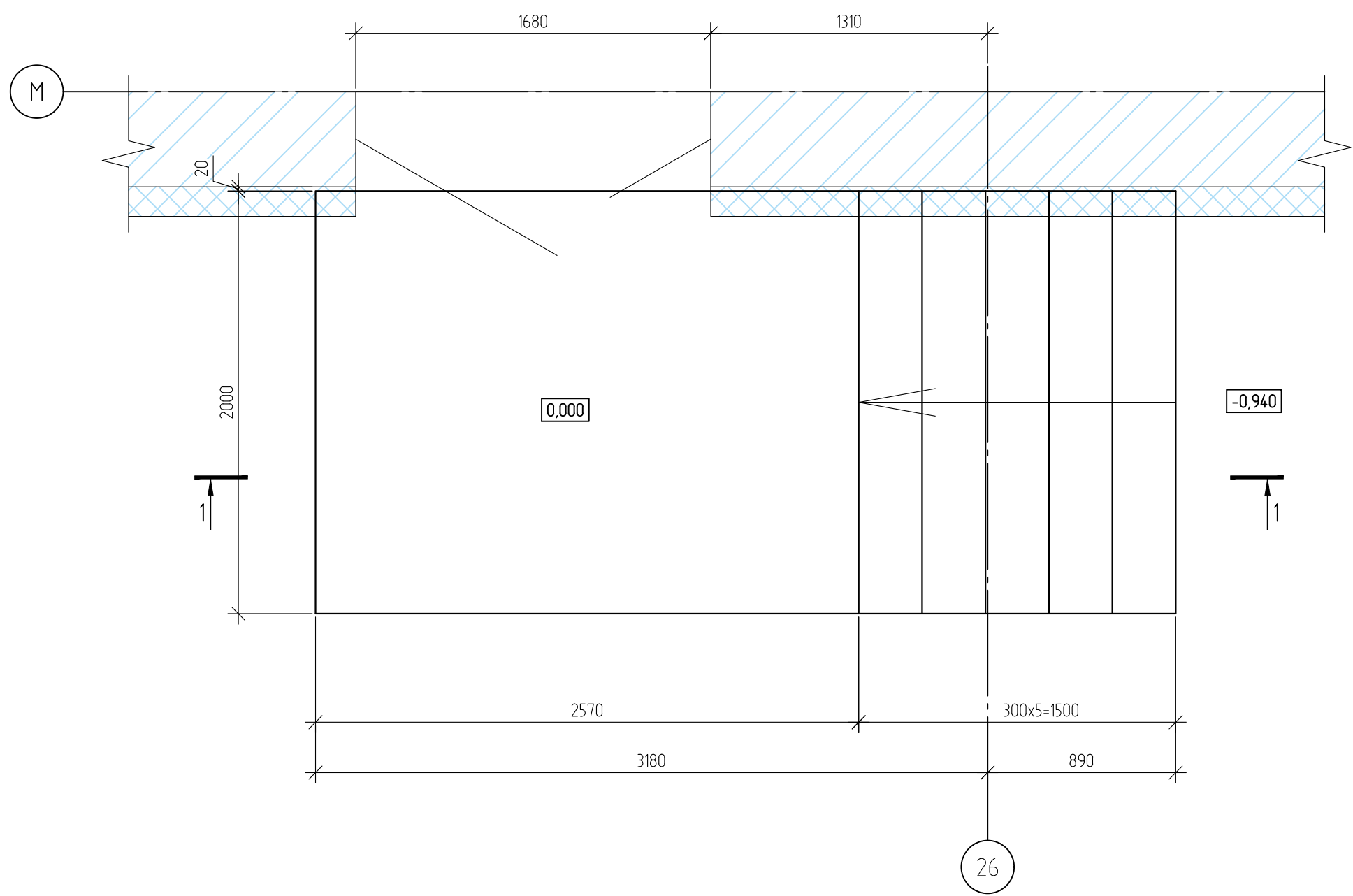
Схема устройства входа в осях "26/М"
