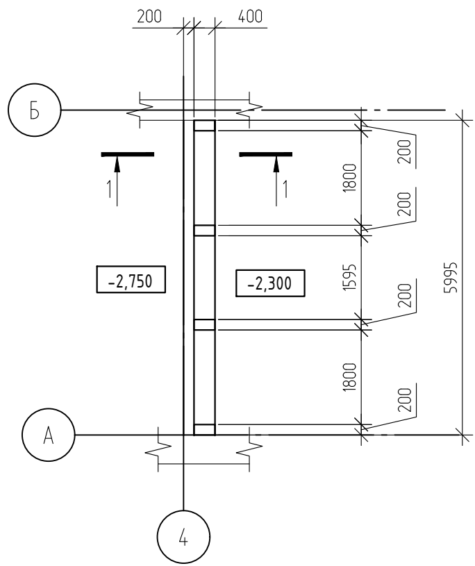
Подпорная стена ПС-1.1
