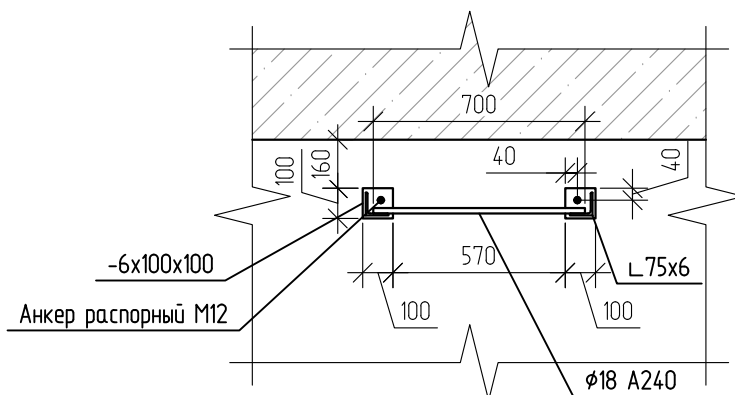
Разрез 2-2
