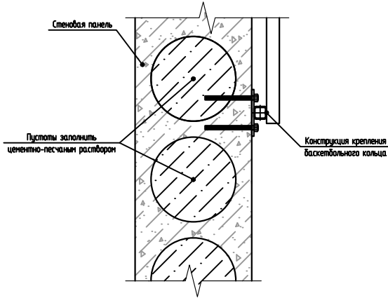
Схемы усиления стен в местах крепления спортивного инвентаря
