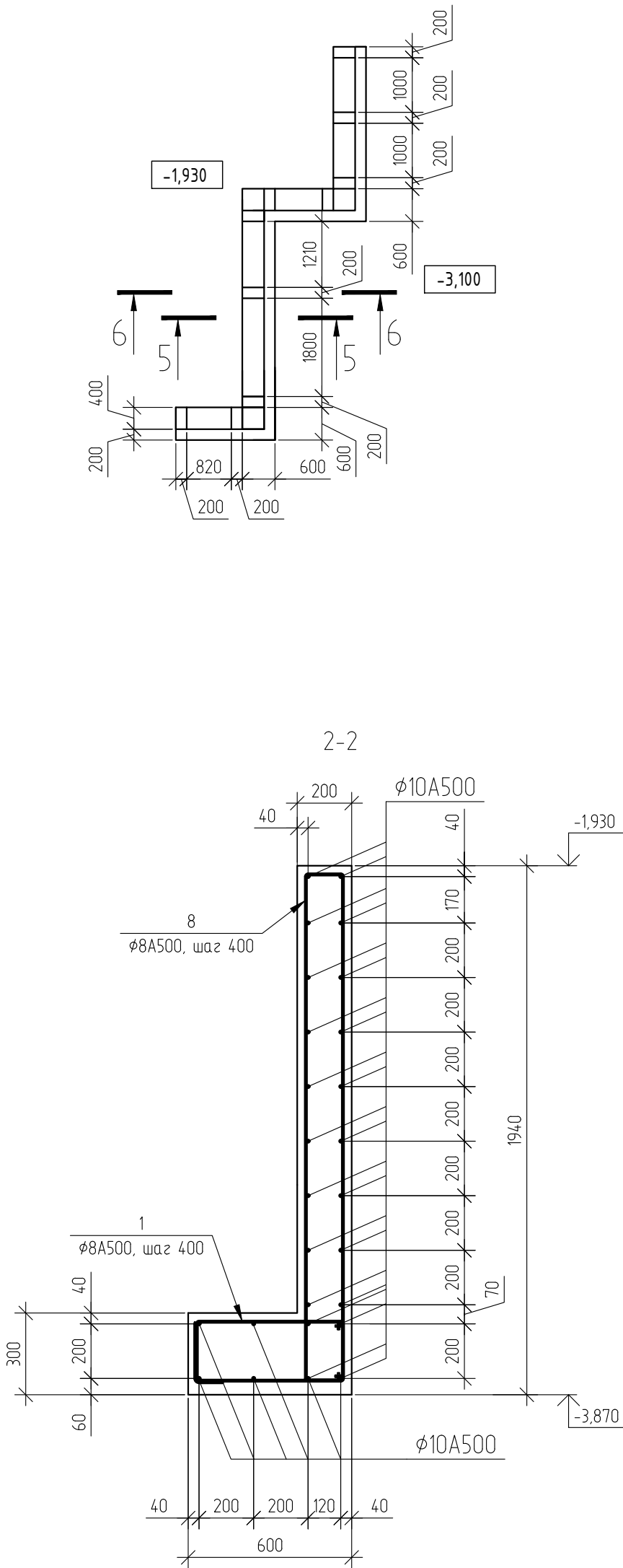
Подпорная стена ПС-1.6
