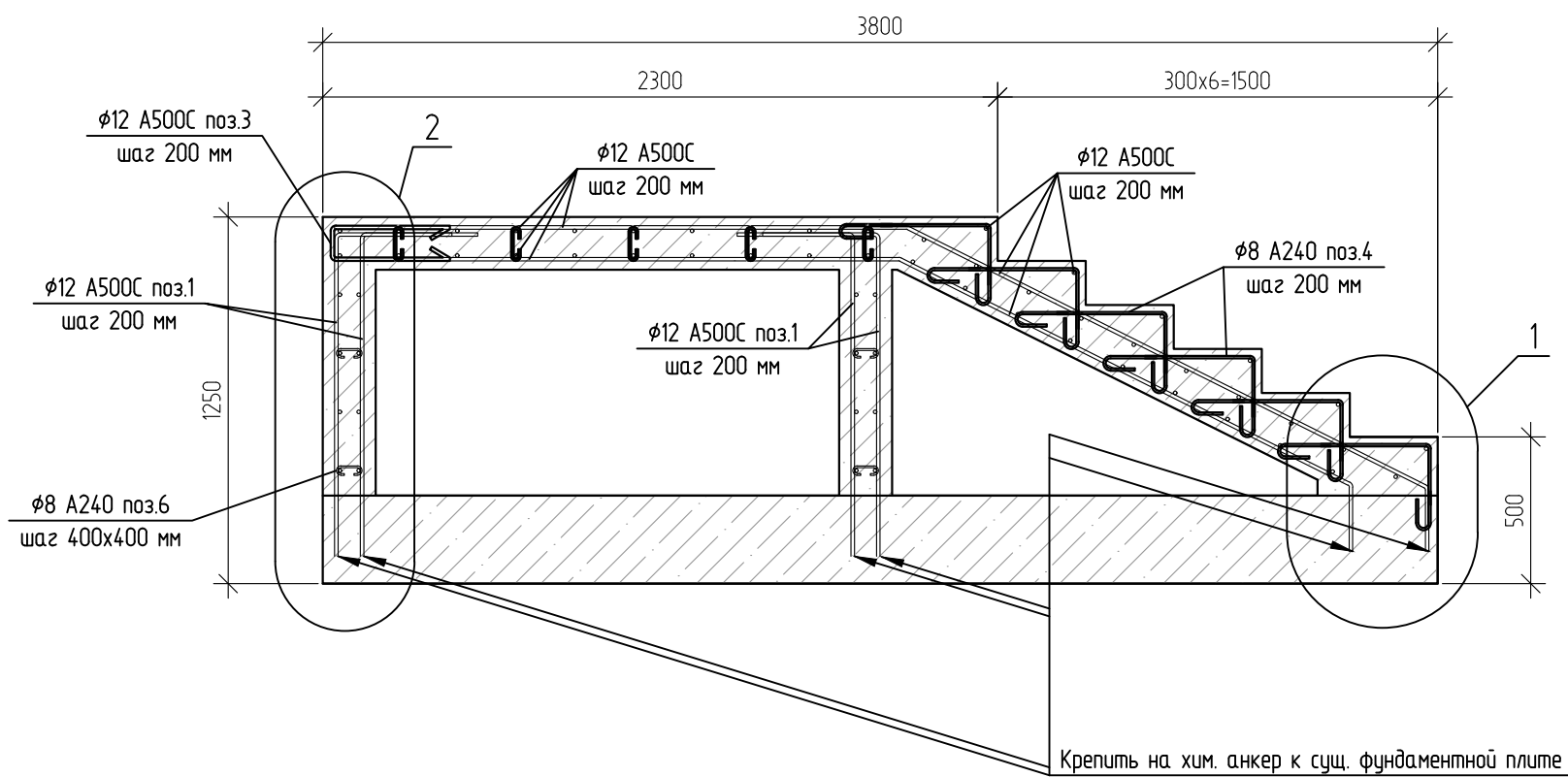
Армирование 1-1
