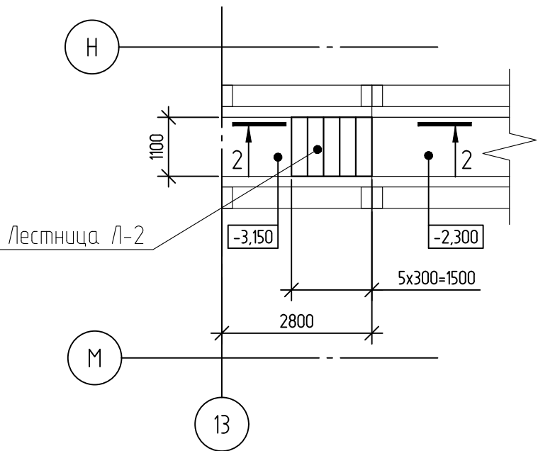
Схема расположения лестницы Л-2
