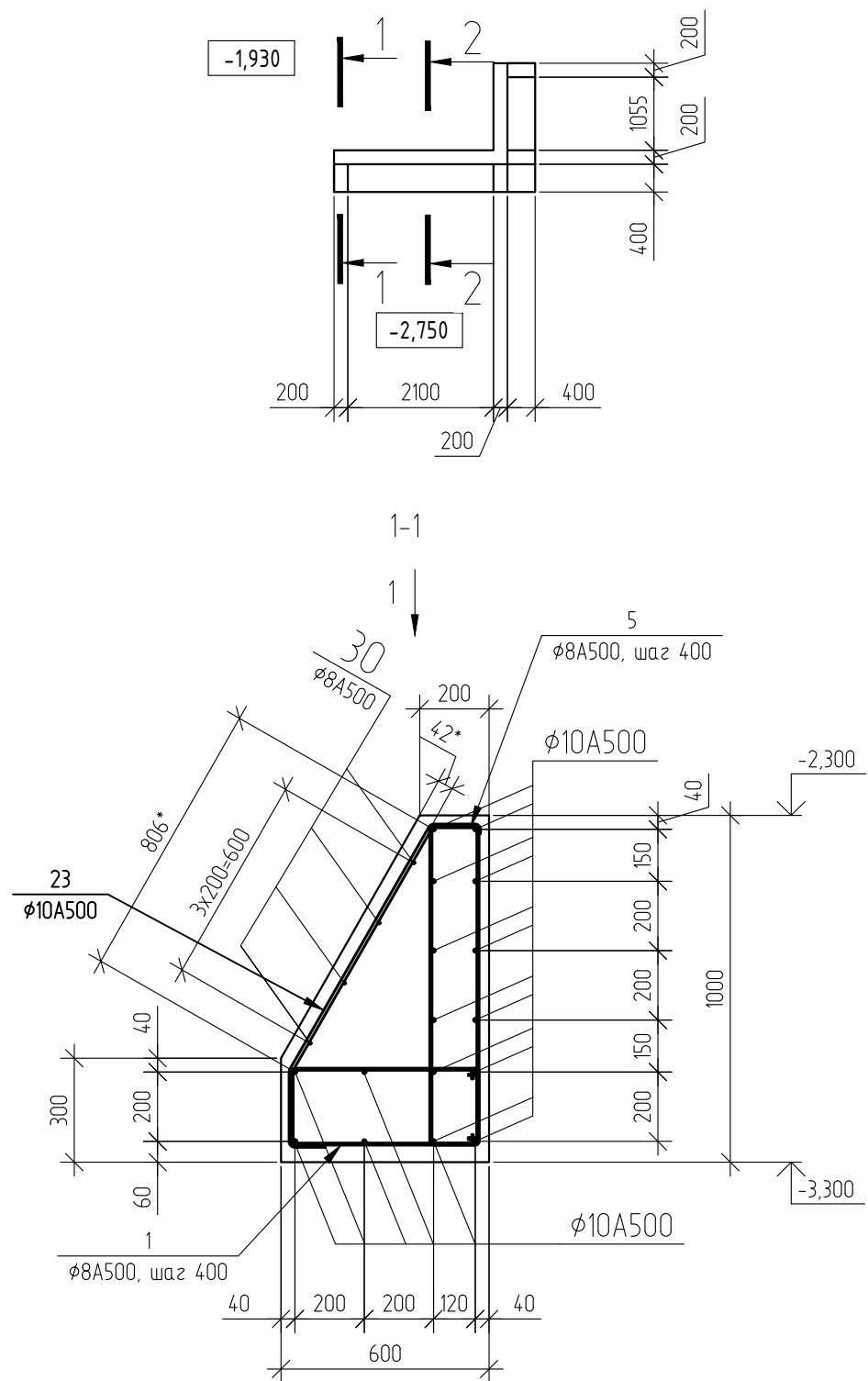
Подпорная стена ПС-1.4
