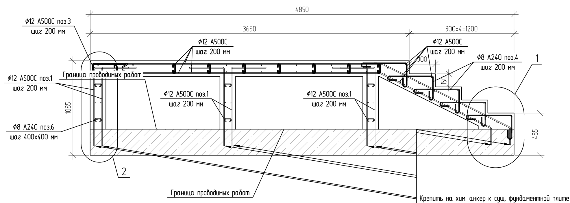
Армирование 1-1
