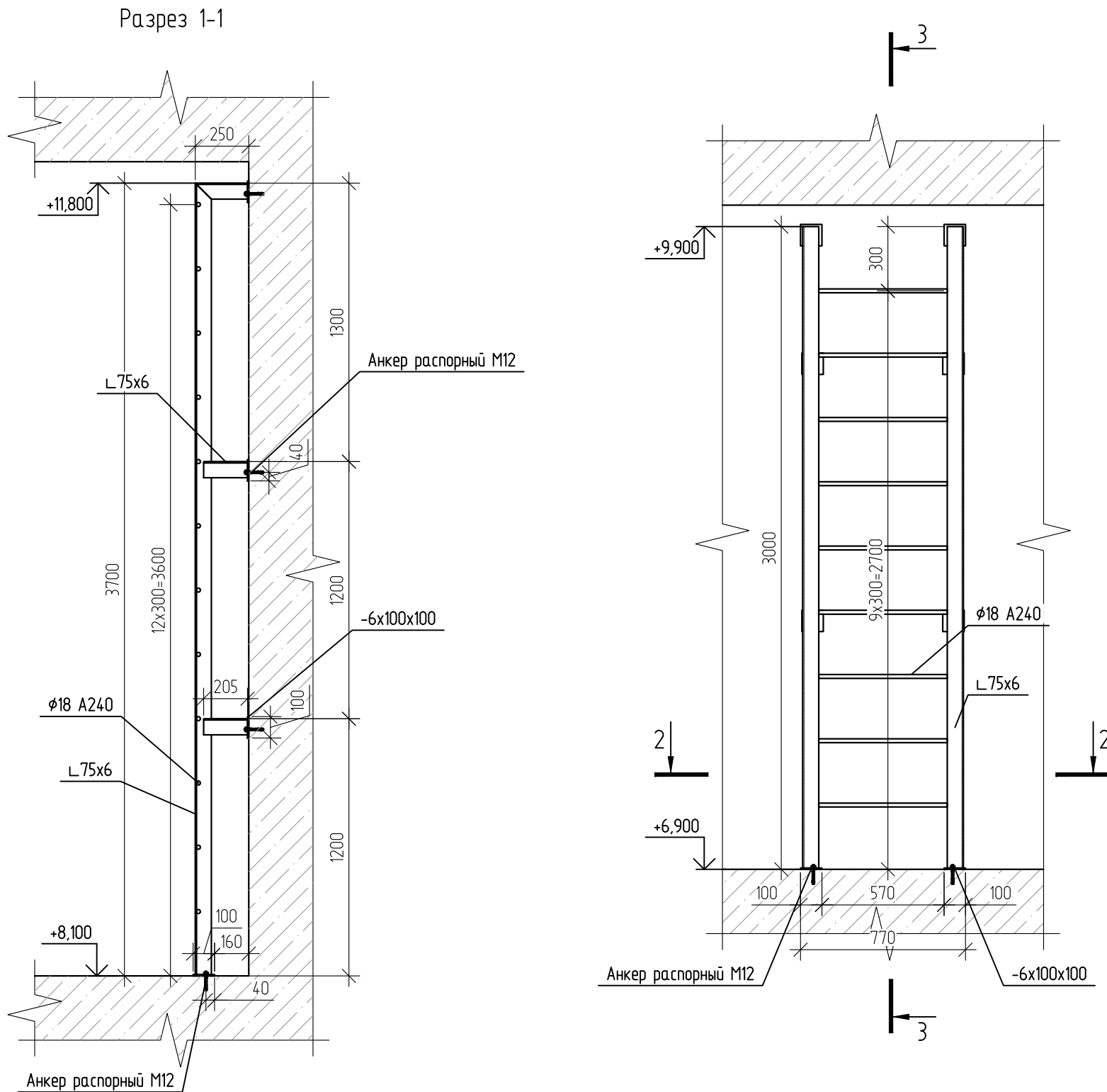
Схема устройства лестницы ПЛ-2
