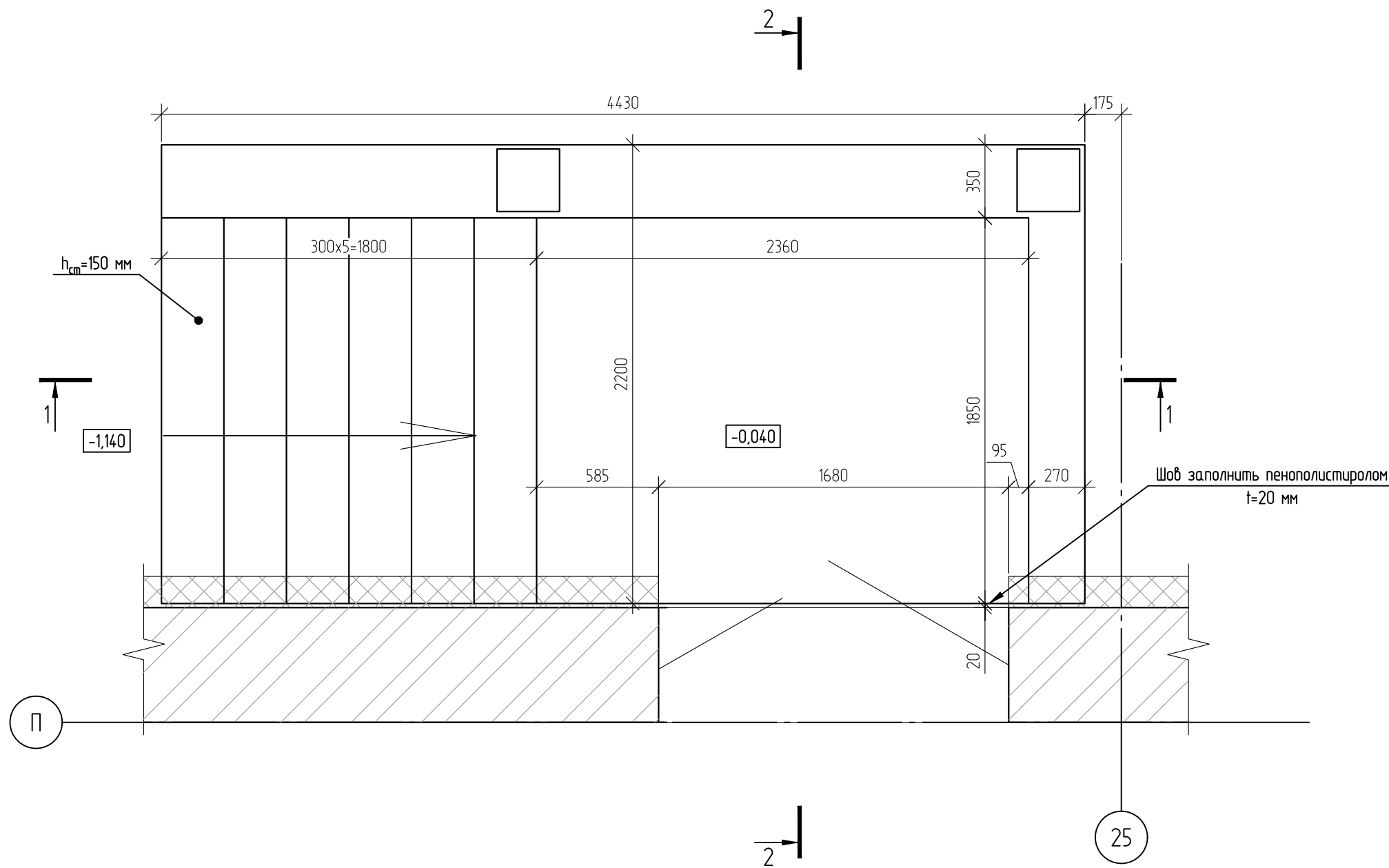
Схема устройства входа в осях "25/П"
