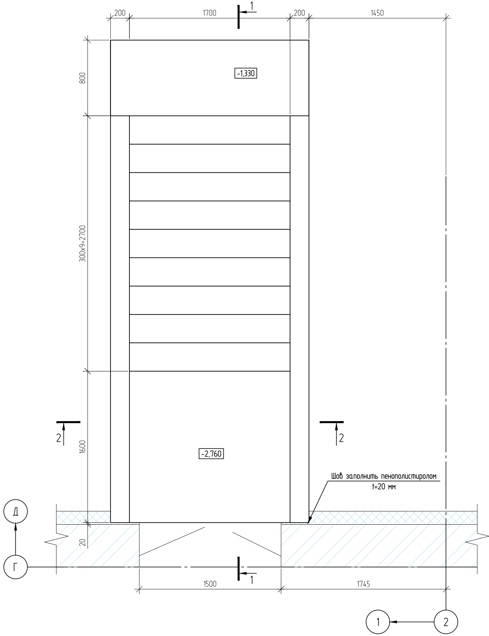
Схема устройства входа в осях "1-2/Г-Д"
