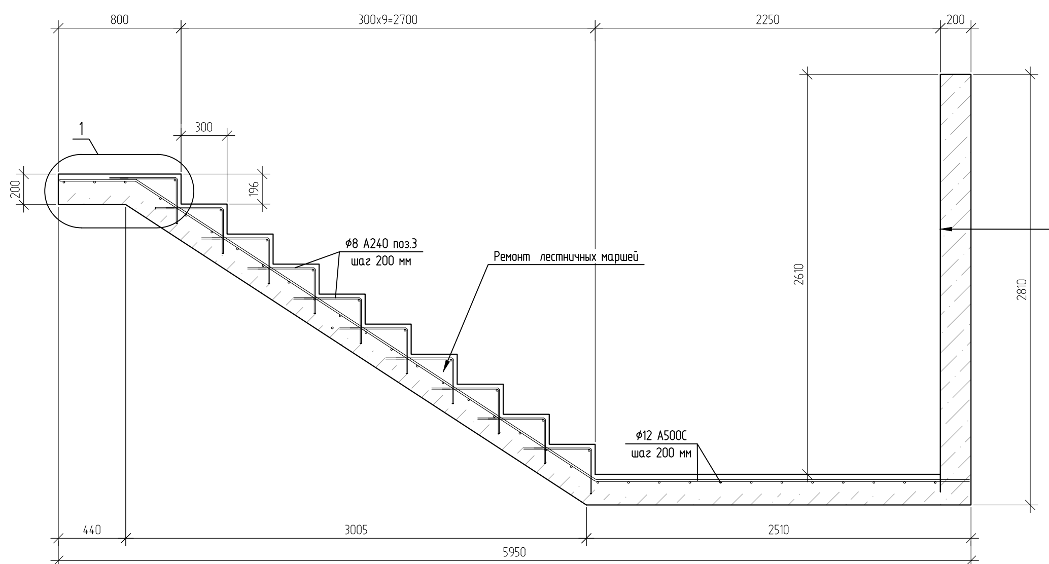
Армирование 1-1
