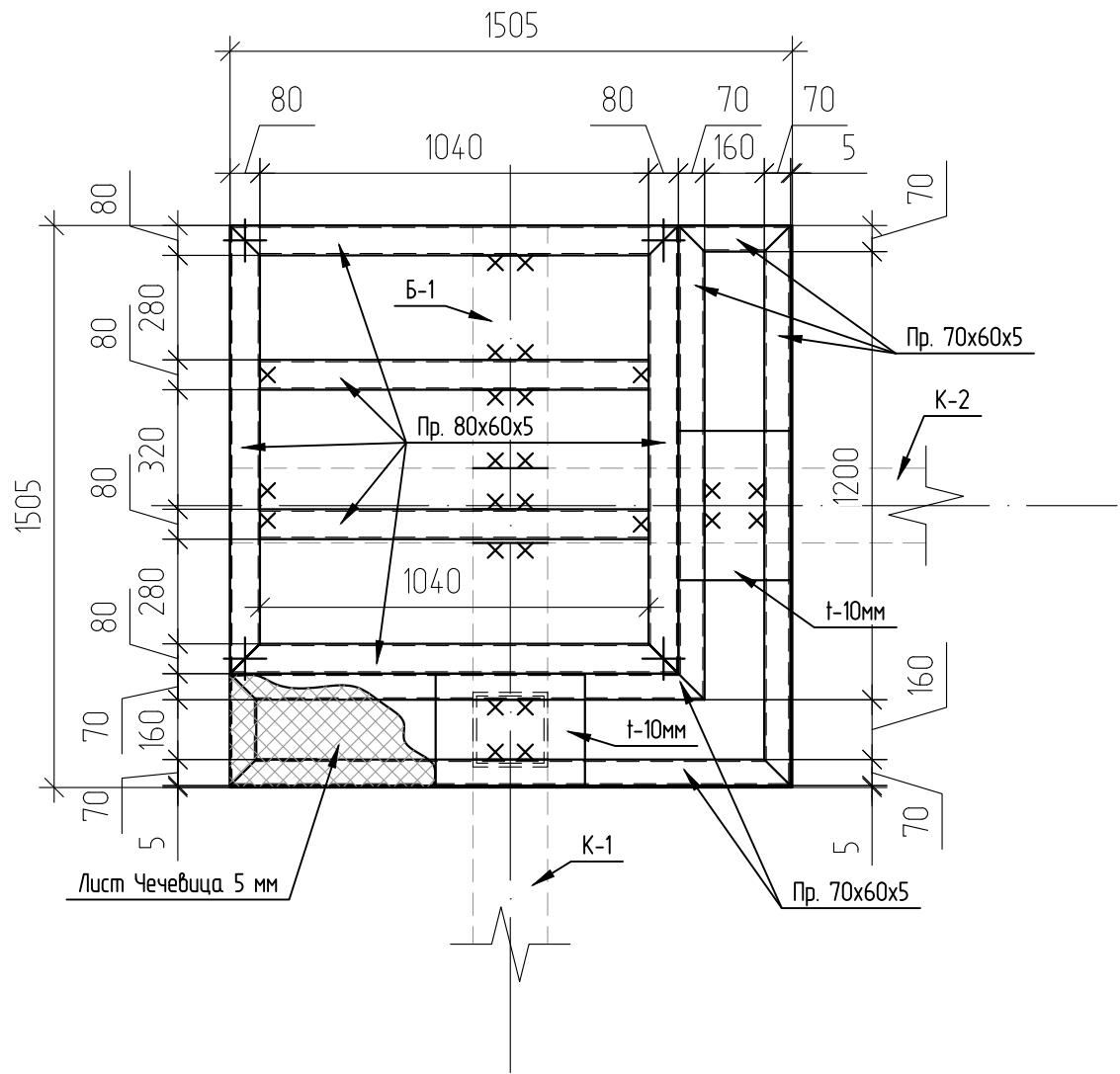
Площадка на отм. +1.220
