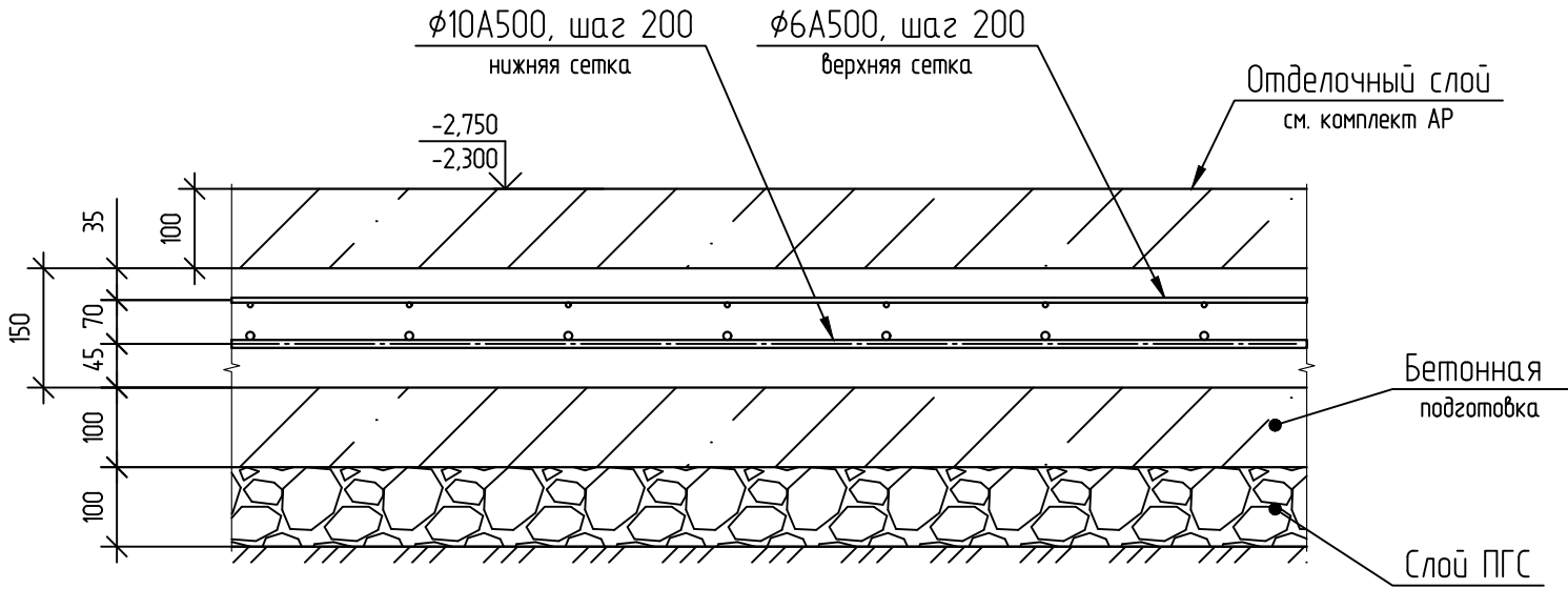
Схема армирования плиты пола подвала ПП-1
