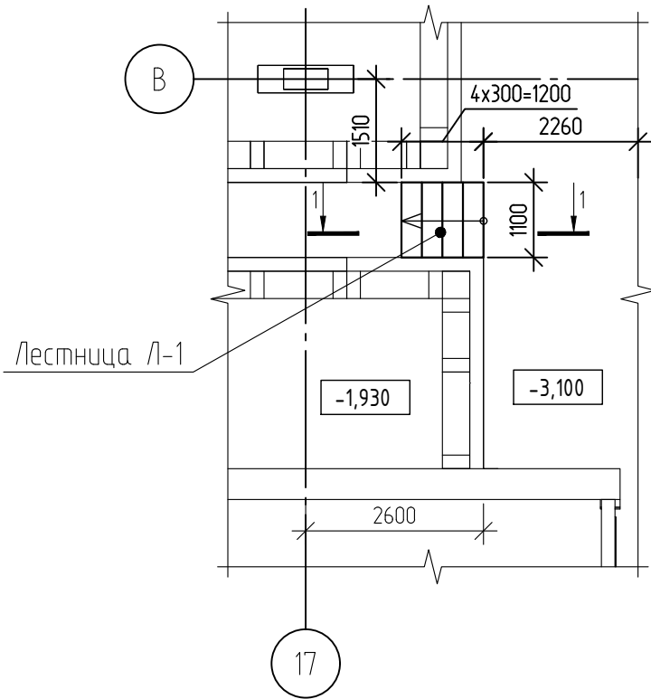
Схема расположения лестницы Л-1
