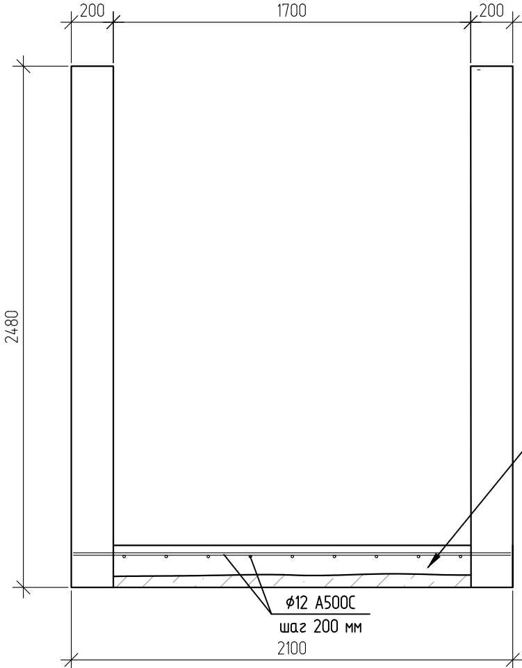
Армирование 2-2
