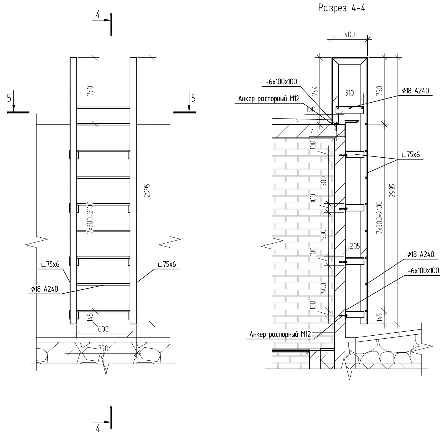
Схема устройства лестницы ПЛ-3
