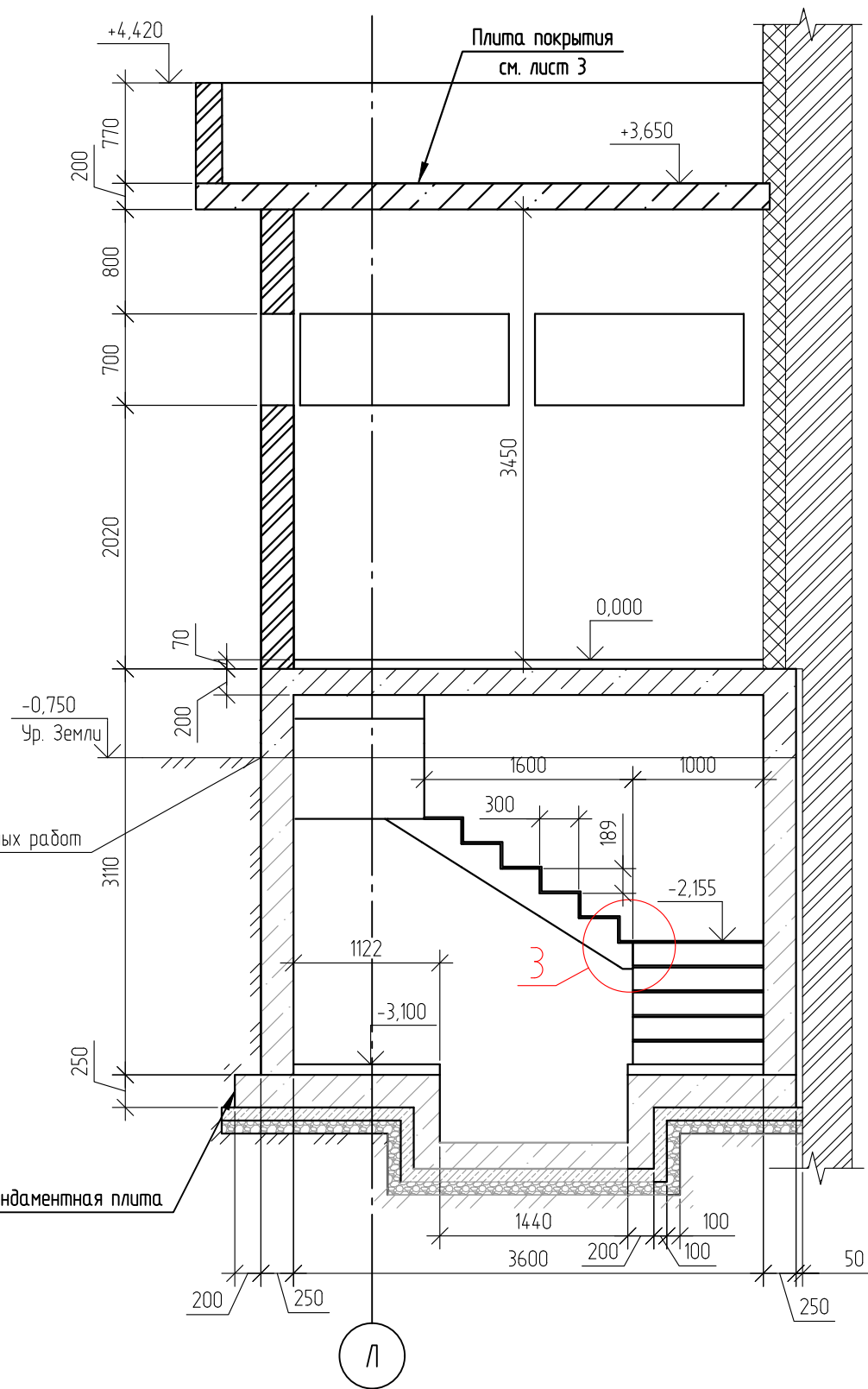
Разрез 2-2
