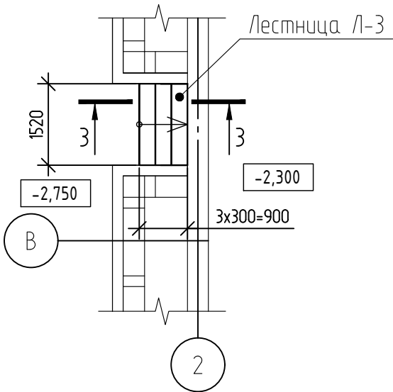
Схема расположения лестницы Л-3
