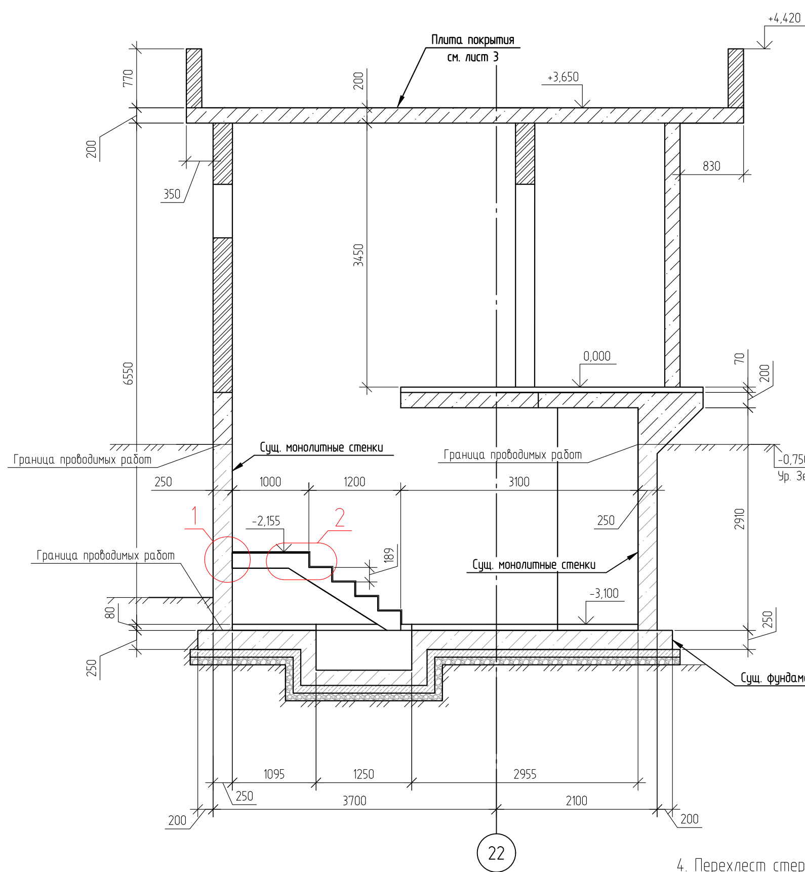
Разрез 1-1
