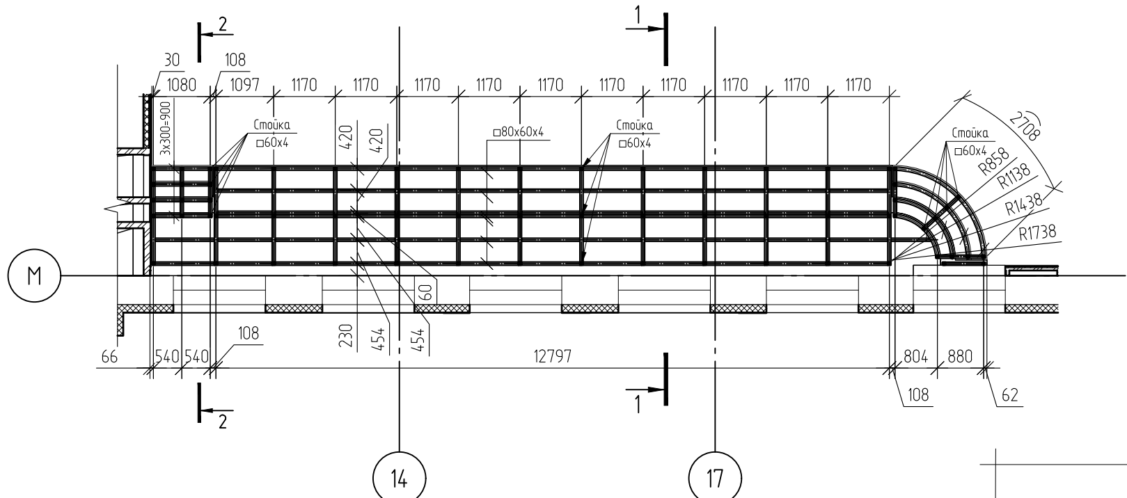
Металлокаркас зрительной трибуны на отм. +3.300 в осях 13-21/М
