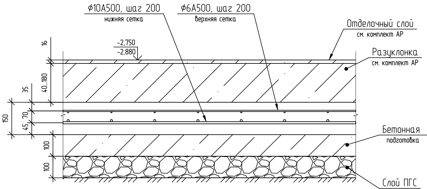
Схема армирования плиты пола подвала ПП-2
