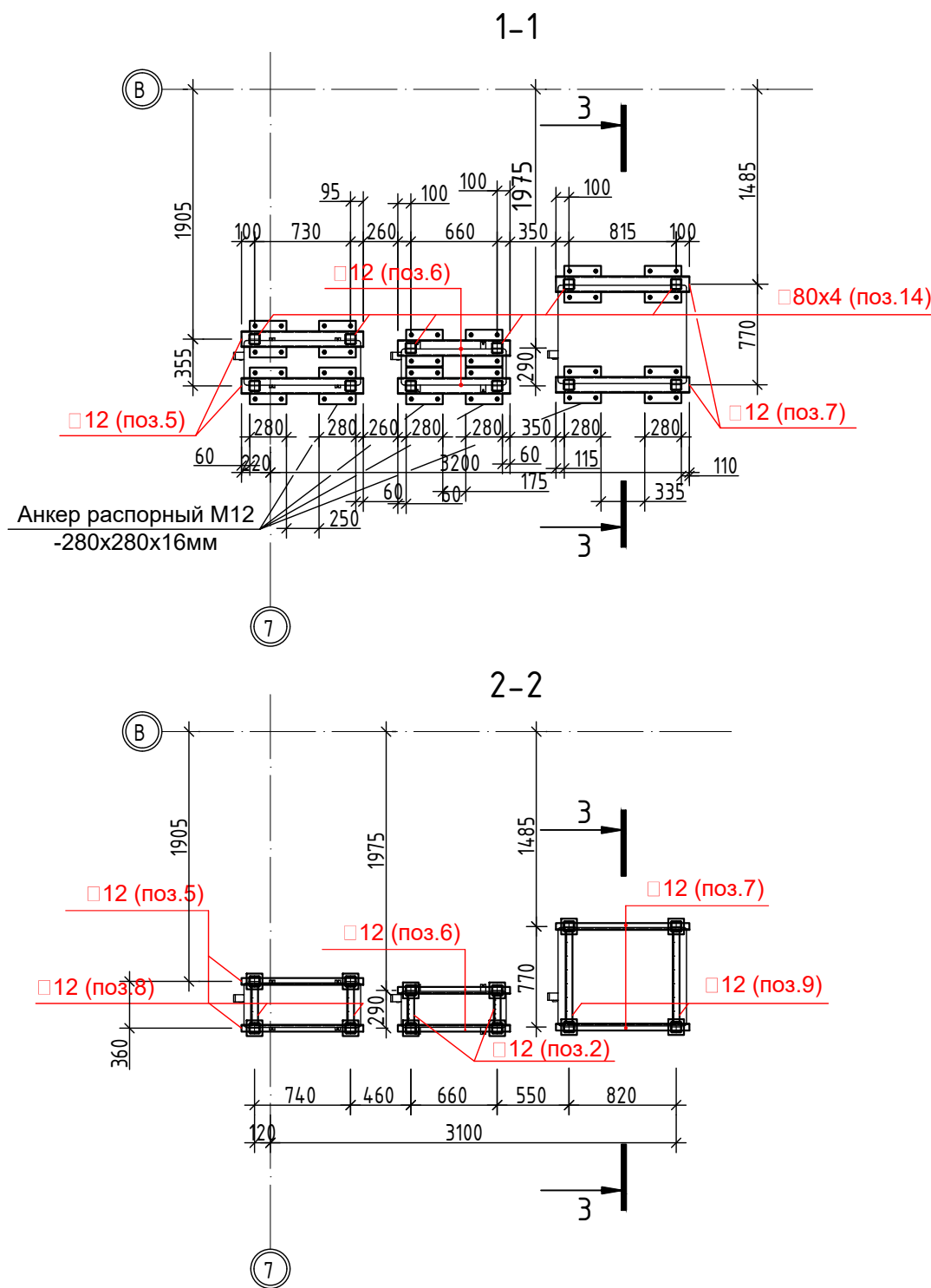
Схема рамы на кровле для оборудования кондиционирования в осях В/7
