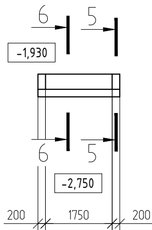
Подпорная стена ПС-1.3
