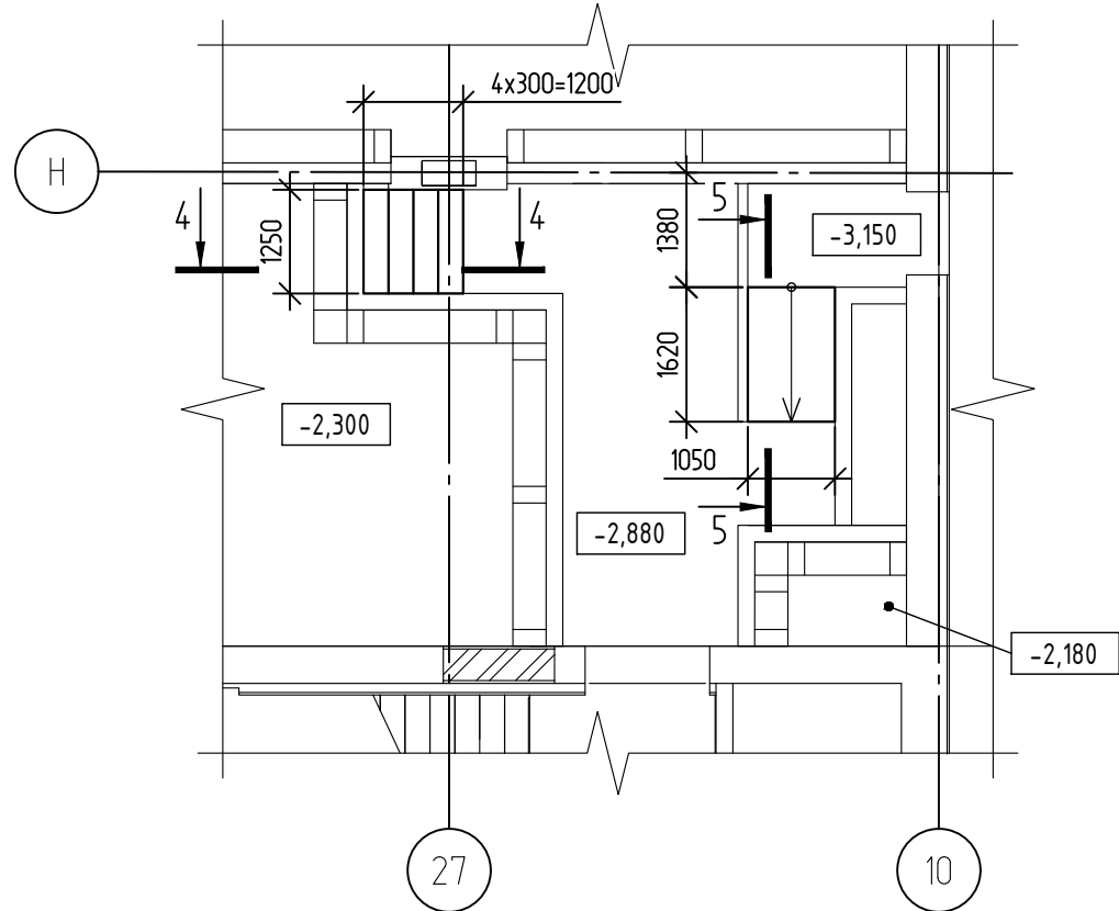
Схема расположения лестницы Л-3 и пандуса П-1
