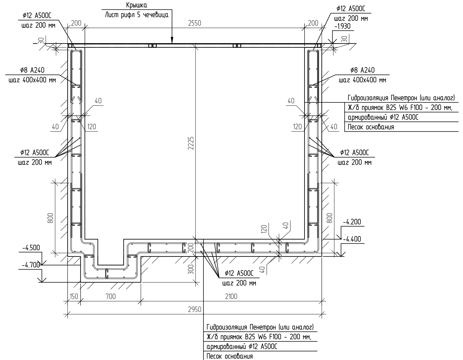
Разрез 1-1
