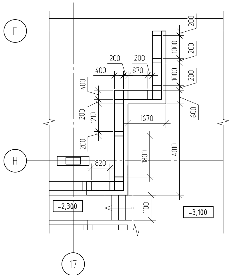
Подпорная стена ПС-1.6
