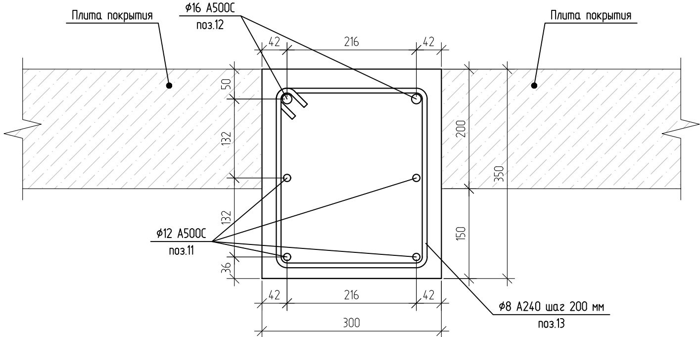
Схема армирования балки покрытия
