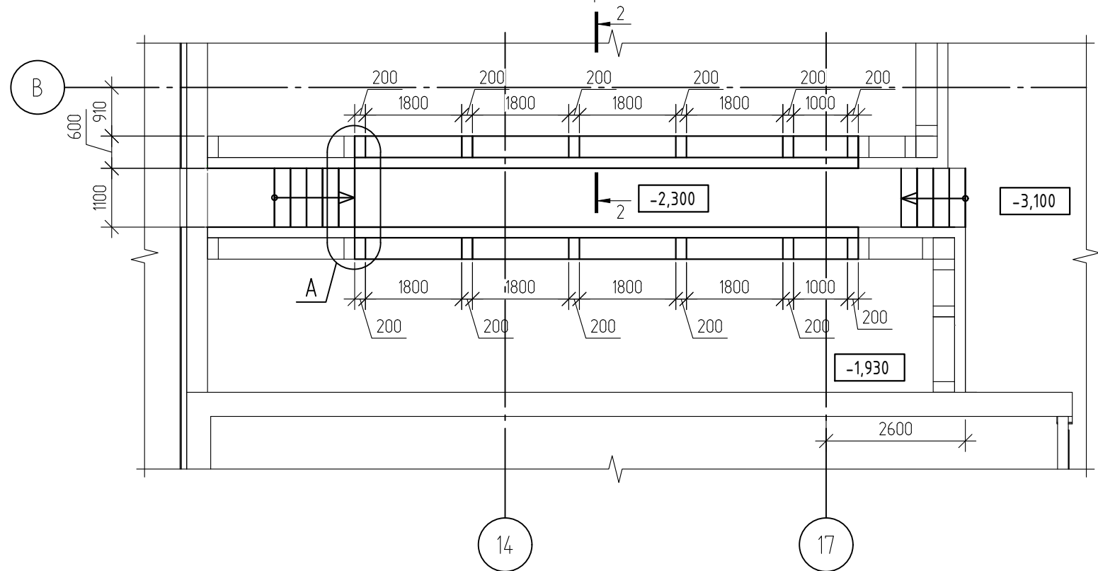
Подпорная стена ПС-1.5
