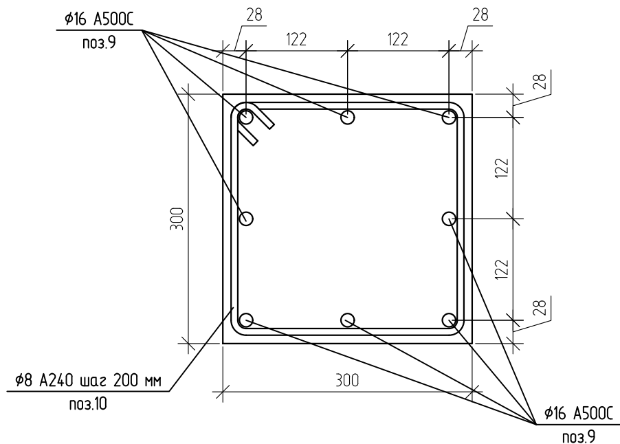
Схема армирования колонны Разрез 5-5
