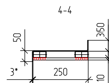
Ступень Ст-1
