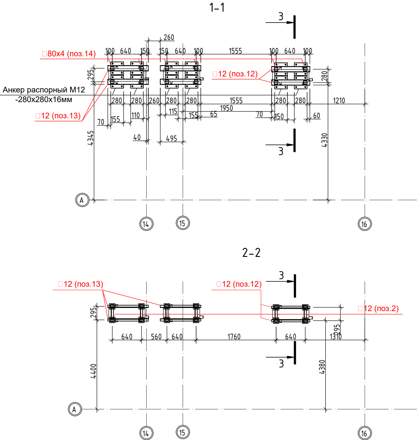
Схема рамы на кровле для оборудования кондиционирования в осях А/14-16
