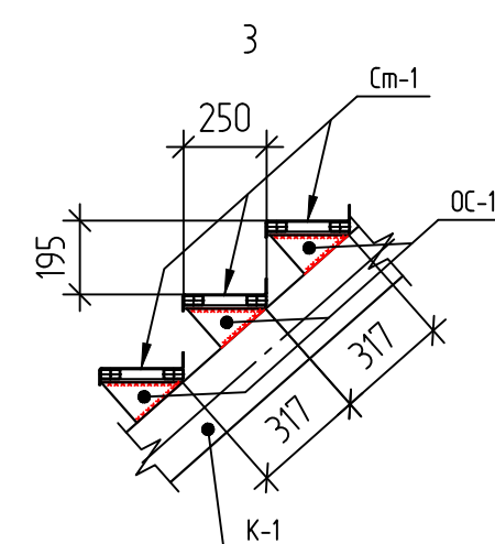
Ступень Ст-1
