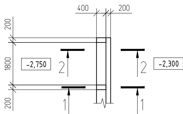
Подпорная стена ПС-1.1 (фрагмент)
