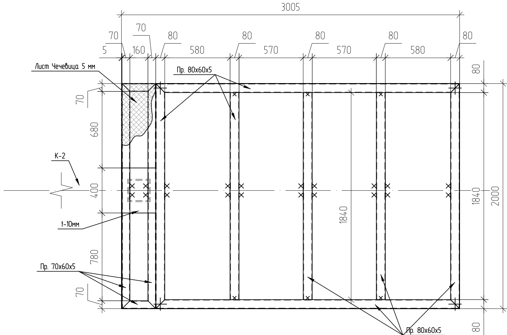
Площадка на отм. +3.300
