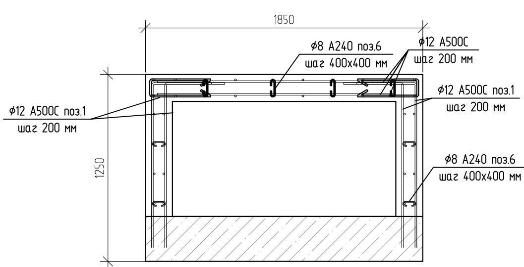
Армирование 2-2
